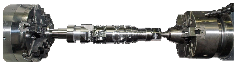
Afbeelding: demo-werkstuk
